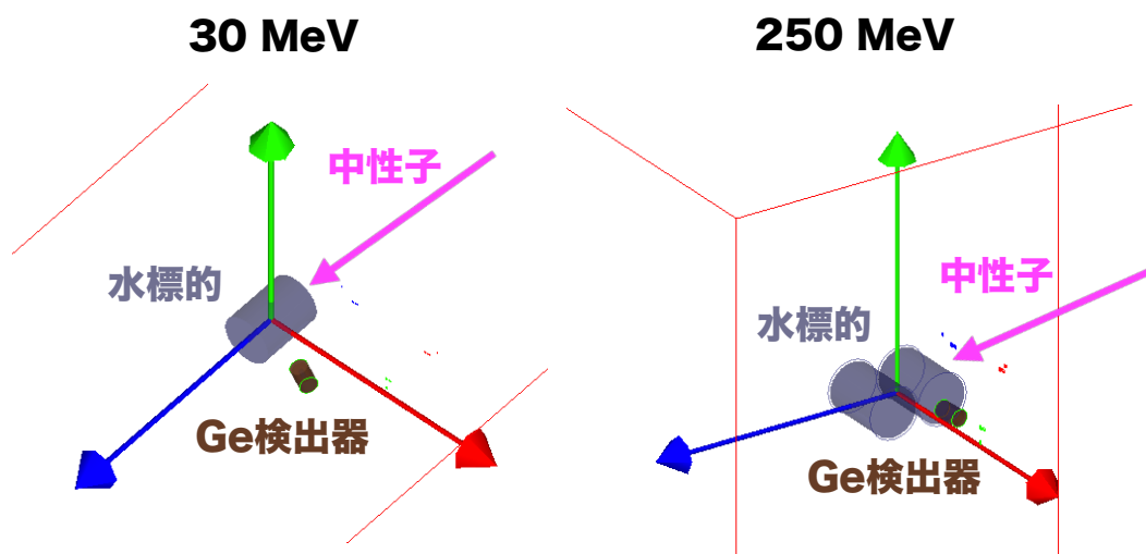
図 7.3: 30 MeV(左)と 250 MeV(右)におけるシミュレーションのセットアップ図。ピンクで示した矢印の方向から中性子ビームを入射する。
