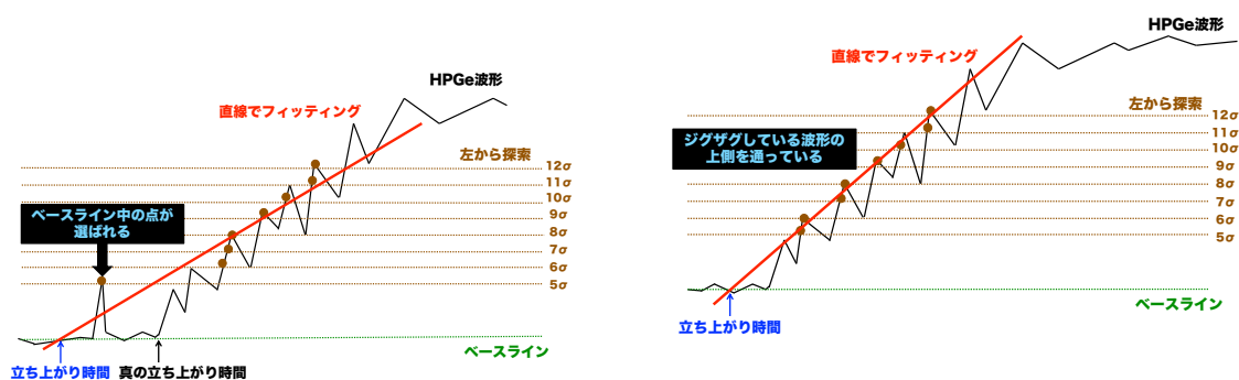
図 5.7: 全ての点を左側から探索していった際の立ち上がり時間計算の様子。 5\sigma - 12\sigma のラインを 図 5.6: ベースライン中に 5\sigma を超える点が存在し立ち上がり時間計算の様子。 5\sigma - 12\sigma のラインを していた場合、立ち上がり時間は真の時間より早く初めて上回る点を取得するため、ジグザグしてい る波形の上側を通る直線になり、真の時間よりも 早く計算される。
