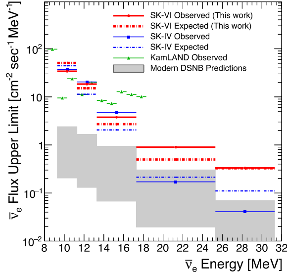
図 1.13: SRN フラックス上限値 [17]. 高い中性子検出効率により, SK-Gd 実験の 552.2 日間のデータを用いた結果は, 純水期の 2970 日間の結果と同等の上限値を与えている.
