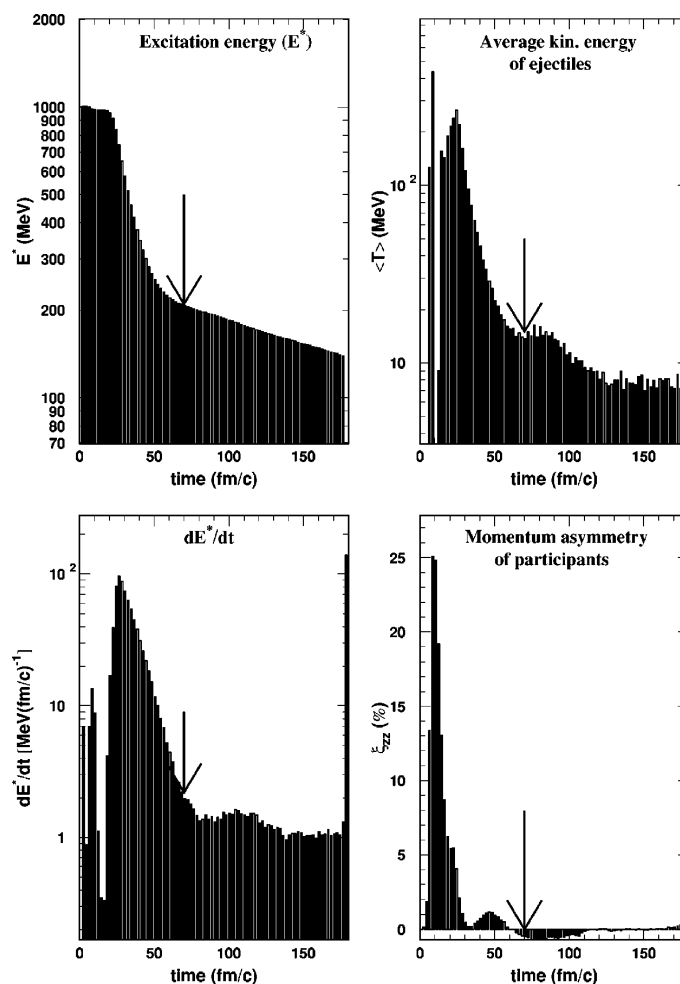
図 7.2: 1 GeV 陽子と鉛の衝突実験における励起エネルギー (左上), 放出核子の平均運動エネルギー (右上), 励起エネルギーの時間微分 (左下), 運動量の非対称性 (右下) の時間変化 [47]. 図中の矢印は t_{stop} の位置を表している.
