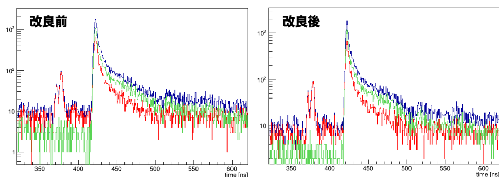
図 4.17: 30 MeV 実験で使用された解析プログラムを用いた場合と本解析で使用したプログラムを用いた場合における、250 MeV 実験の ToF 分布
