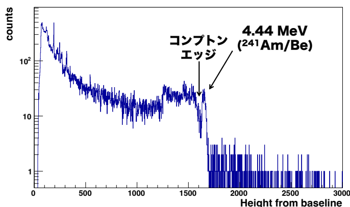
図 5.10: ^{241}\text{Am}/\text{Be} 線源と ^{56}\text{Fe} を用いた測定における波高分布. コンプトンエッジと 4.44 MeV の光電吸収ピークが確認できる. ^{56}\text{Fe} 由来のピークは統計が不十分のため確認することができなかった.
