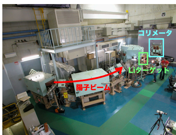
図 3.5: N0 コースにおける中性子生成の様子. {}^7\text{Li}(p, n){}^7\text{Be}^* 反応によって生成された中性子はコリメータを通過して 100 m トンネルへと入射する.
