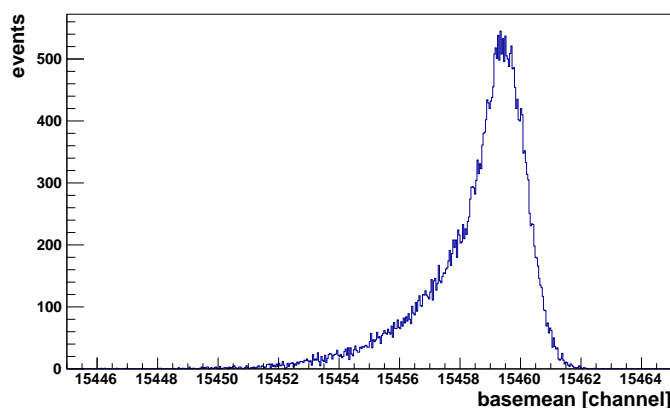
図 4.4: 計算されたベースラインの分布. 良い精度でベースラインを求められている。
