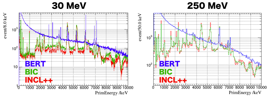
図 7.4: 30 MeV(左) と 250 MeV(右) におけるモデル毎のガンマ線スペクトル. 青が BERT, 緑が BIC, 赤が INCL++を表す. このスペクトルをエネルギー分解能曲線で鈍らせ, 検出器の応答を考慮する.
