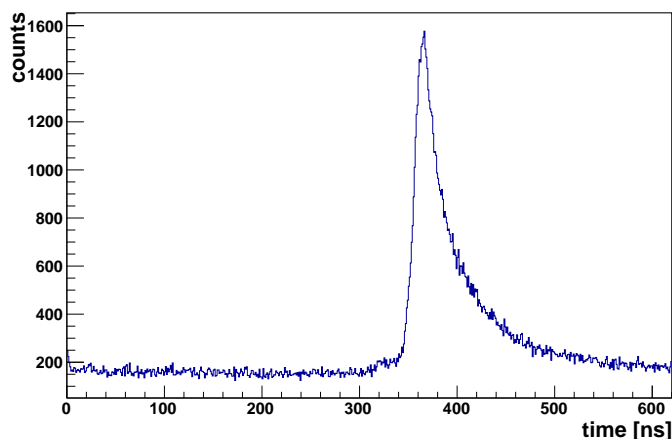
図 5.15: HPGe 検出器における ToF 分布。ビーム軸上に置かれていないため、即発ガンマ線のピークは見られていない。
