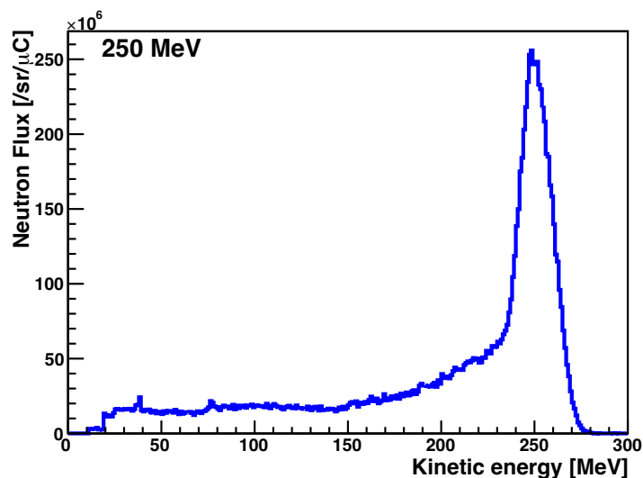
図 4.22: 中性子フラックス分布
