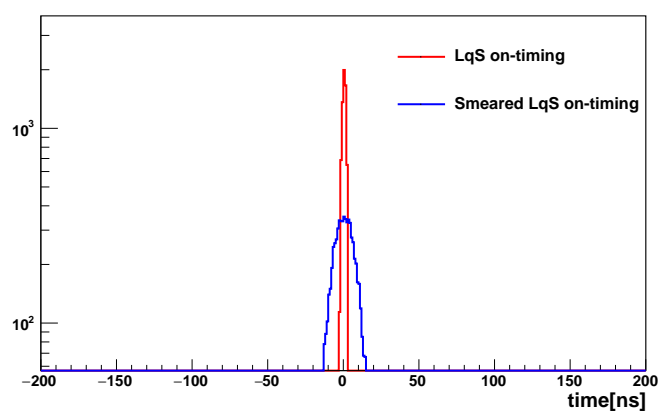
図 5.18: BC-501A の On-timing 領域における ToF 分布 (赤色) とそれを時間分解能 6.8 ns に鈍らせた分布 (青色).
