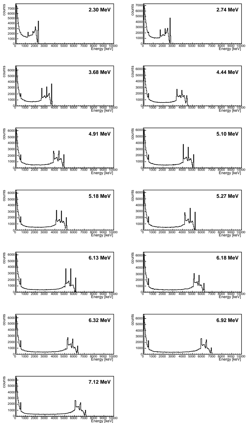
図 5.25: 用意したシグナルテンプレート
